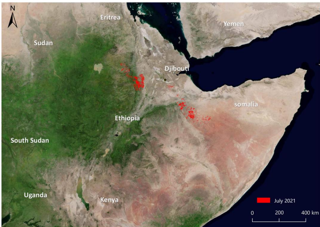
图 3 埃塞俄比亚沙漠蝗虫危害区域遥感监测图（2021 年 7 月）
