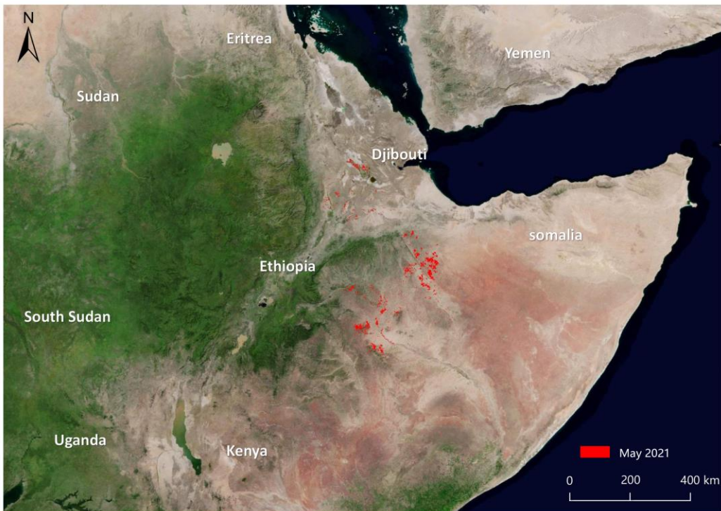
图1 埃塞俄比亚沙漠蝗虫危害区域遥感监测图（2021年5月）
