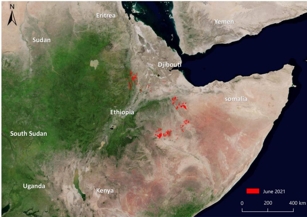
图 2 埃塞俄比亚沙漠蝗虫危害区域遥感监测图（2021 年 6 月）
