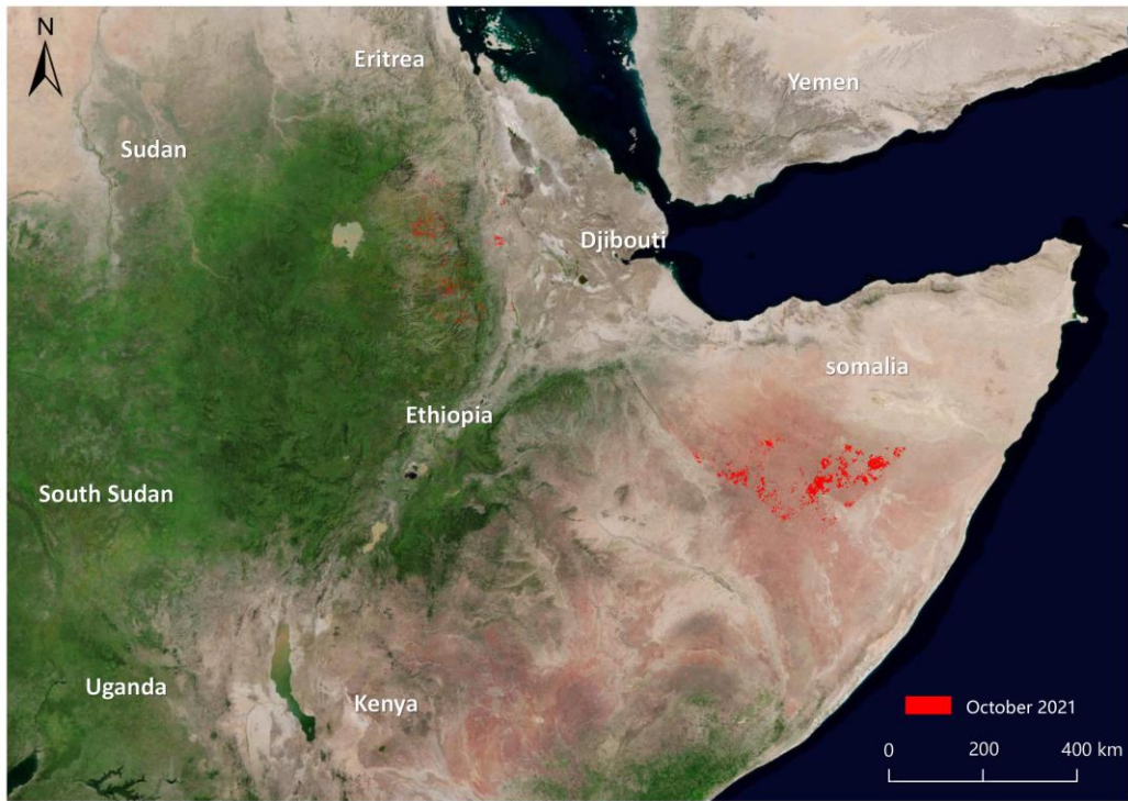
图 2 埃塞俄比亚沙漠蝗虫危害区域遥感监测图（2021 年 10 月）
