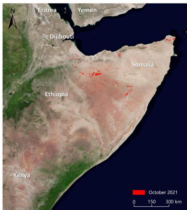
图 1 索马里沙漠蝗虫危害区域遥感监测图（2021 年 10 月）
