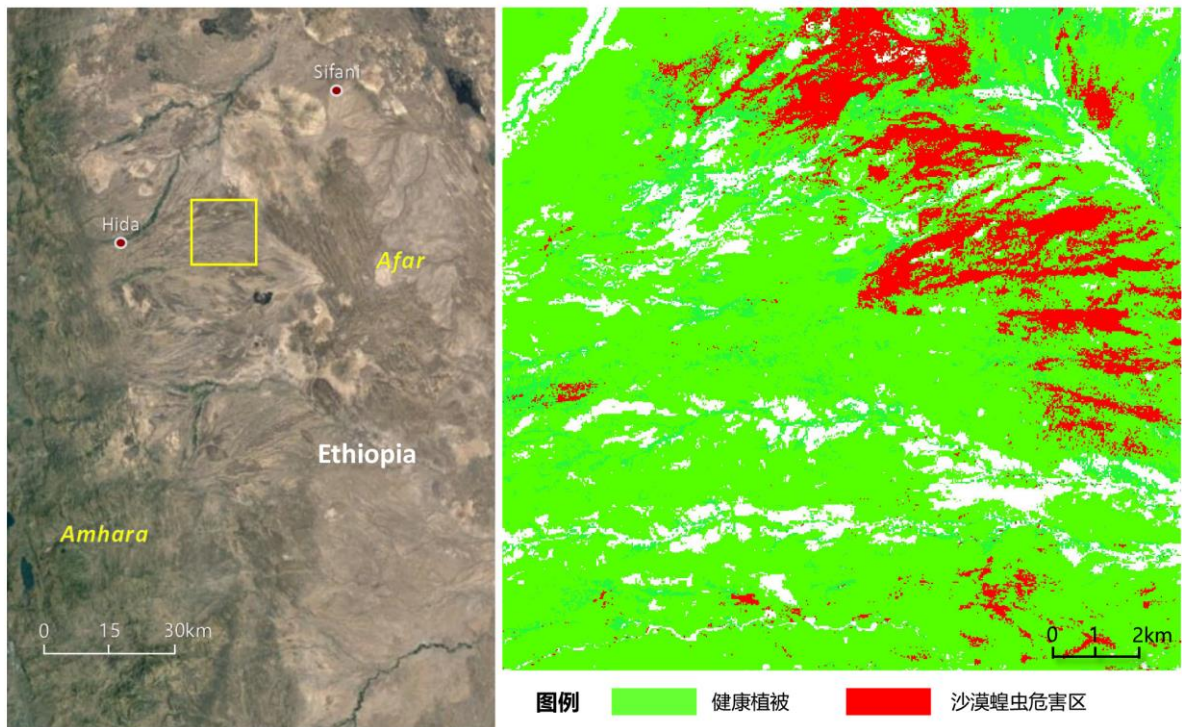
图 3 基于 Sentinel 影像的埃塞俄比亚沙漠蝗虫重点危害区灾害遥感监测（2021 年 10 月）
