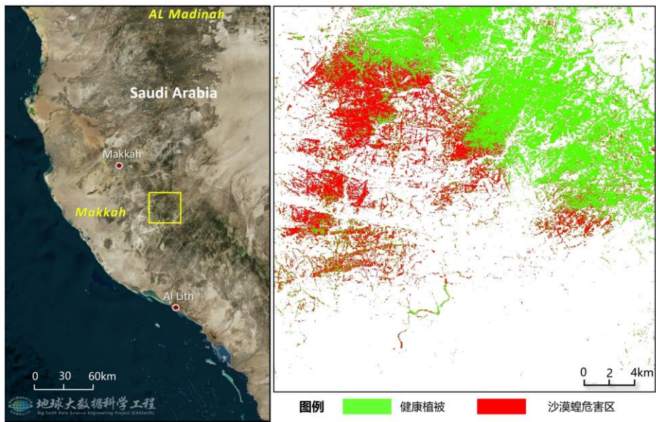
图 3. 基于 Sentinel-2 影像的沙特阿拉伯沙漠蝗重点危害区灾害遥感监测（2023 年 5 月）
