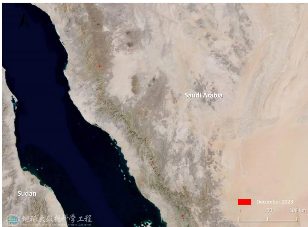
图1. 沙特阿拉伯沙漠蝗危害区域遥感监测图（2023年12月）
