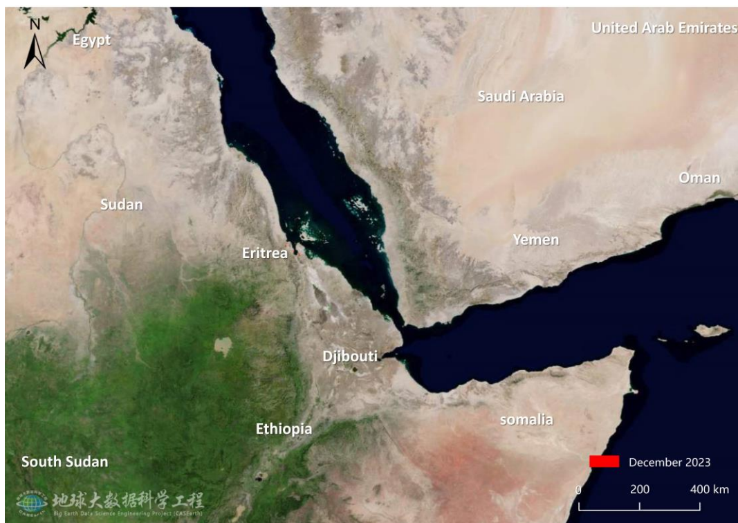
图 2. 厄立特里亚沙漠蝗危害区域遥感监测图（2023 年 12 月）
