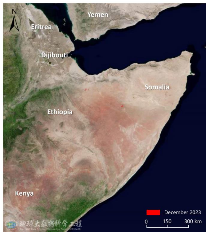
图 3. 索马里沙漠蝗危害区域遥感监测图（2023 年 12 月）
