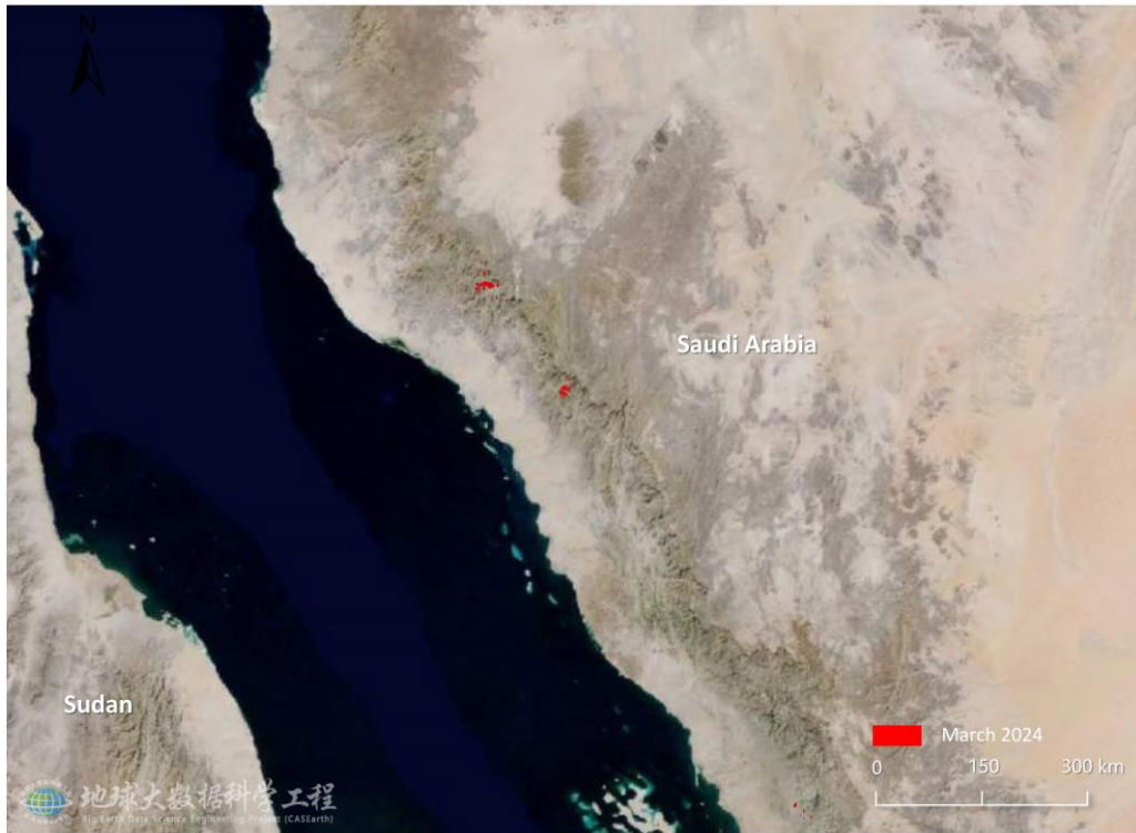
图 1. 沙特阿拉伯沙漠蝗危害区域遥感监测图（2024年3月）
