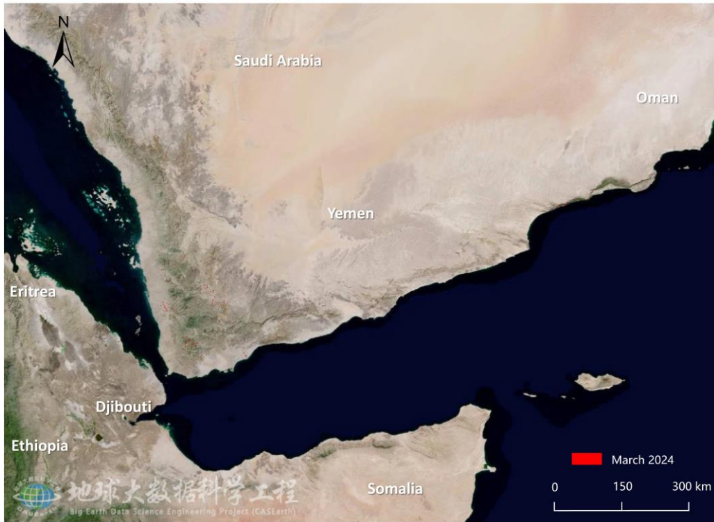
图 2. 也门沙漠蝗危害区域遥感监测图（2024 年 3 月）
