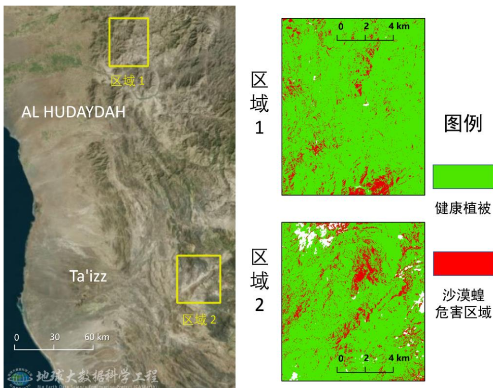
图 3 基于 SDGSAT-1 影像的也门沙漠蝗重点危害区遥感监测（2024 年 3 月）
