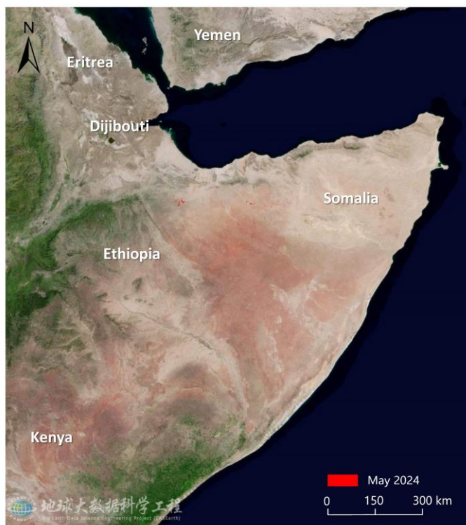
图 1. 索马里沙漠蝗危害区域遥感监测图（2024年5月）
