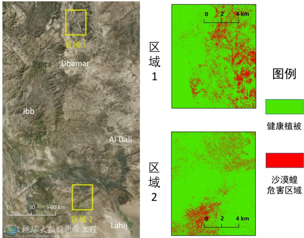
图 3. 基于 Sentinel-2 影像的也门沙漠蝗重点危害区遥感监测（2024 年 5 月）
