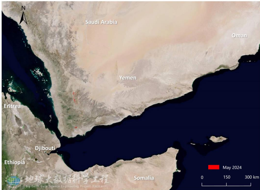
图 2. 也门沙漠蝗危害区域遥感监测图（2024 年 5 月）
