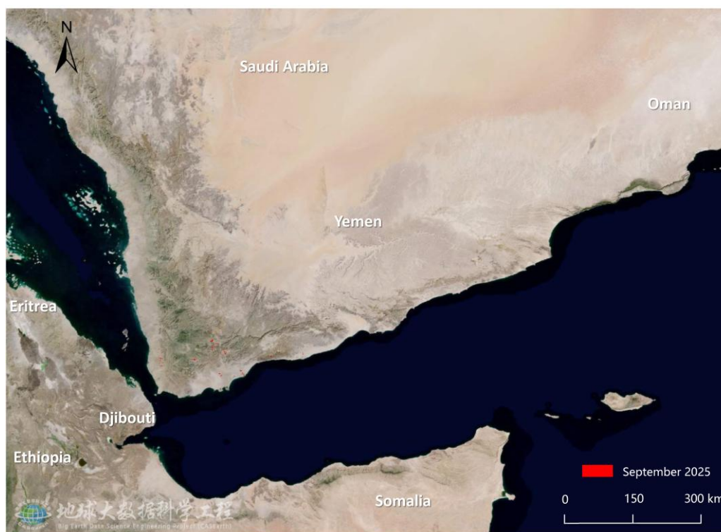
图 3. 也门沙漠蝗危害区域遥感监测图（2025 年 9 月）
