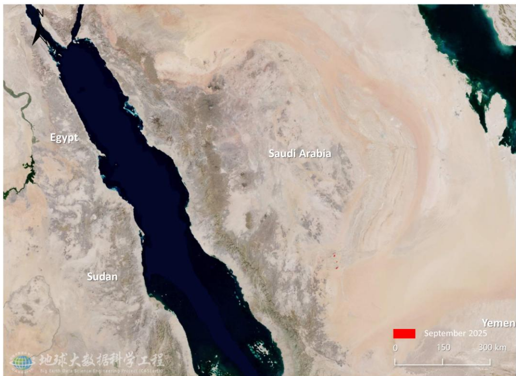
图 2. 沙特阿拉伯沙漠蝗危害区域遥感监测图（2025 年 9 月）
